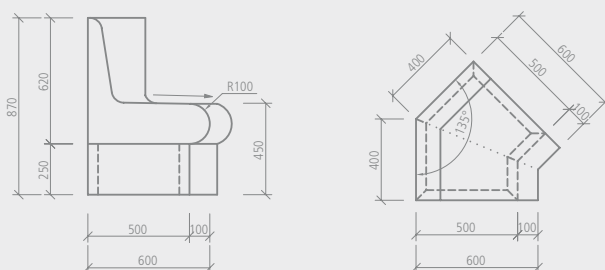
Hjørneelement med lige overgang
