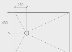
Teknisk tegning Afløbsplacering ved 1200 x 900 mm
