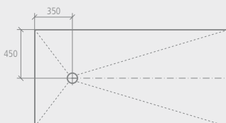
Afløbsplacering ved 1800 x 900 mm
