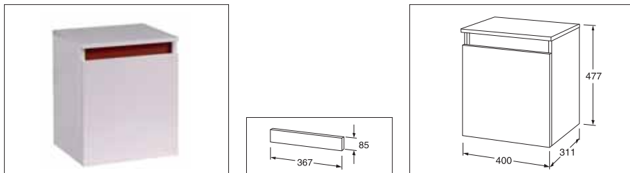
Nautic A669/A670 i hvid højglans med rød pynteliste.
