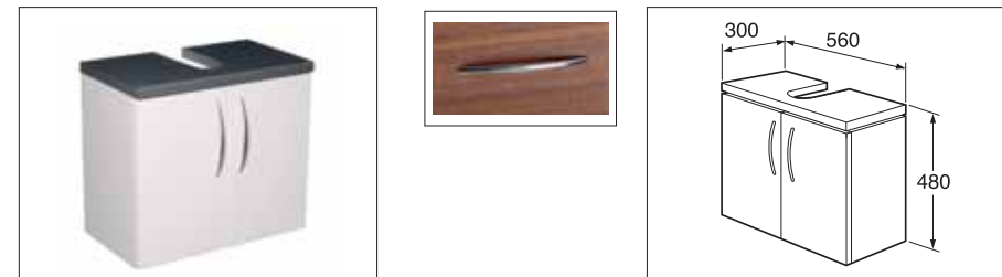
Logic 1856 med gråmeleret bordplade og låger i hvid melamin.
