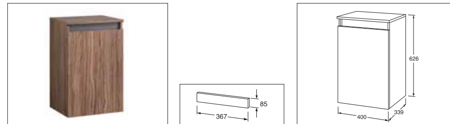
Nautic A667/A668 i oliventræslook med pynteliste i samme farve.
